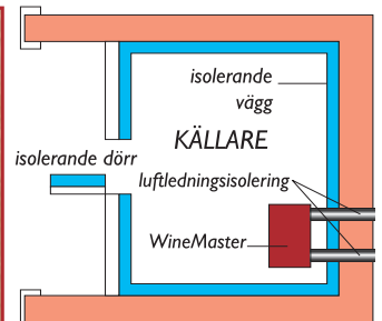
Installationsprincip för IN 50
