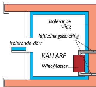
Installationsprincip för IN 18
