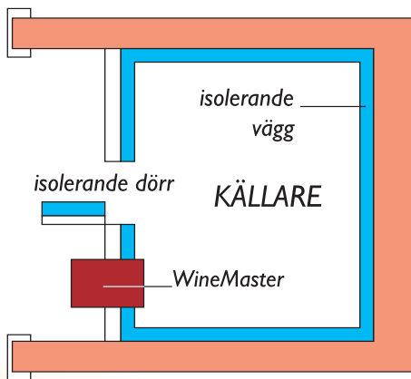
Principinstallation för Wine C
